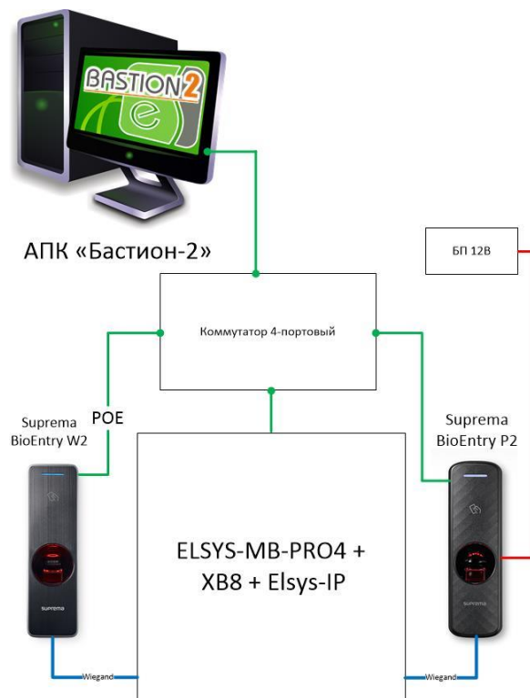
Рис. 1. Пример подключения контроллеров Suprema
